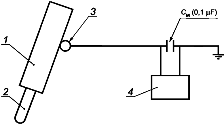
1 — испытательный образец с накопленным зарядом; 2 — тефлоновая ручка; 3 — сферический электрод диаметром (25 \pm 5) мм; 4 — вольтметр диапазоном измерения от 1 до 10 В, соприкасающийся с заряженной поверхностью
