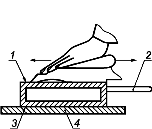
1 — поверхность самой большой площади, подвергающаяся воздействию в любой плоскости; 2 — тефлоновая ручка (или щипцы для перемещения испытательного образца, если используют плоскую пластину); 3 — противоположная поверхность; 4 — изолятор из политетрафторэтилена
